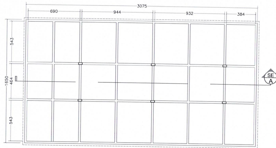
FRAME-2
