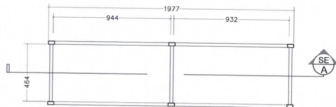
FRAME-1
