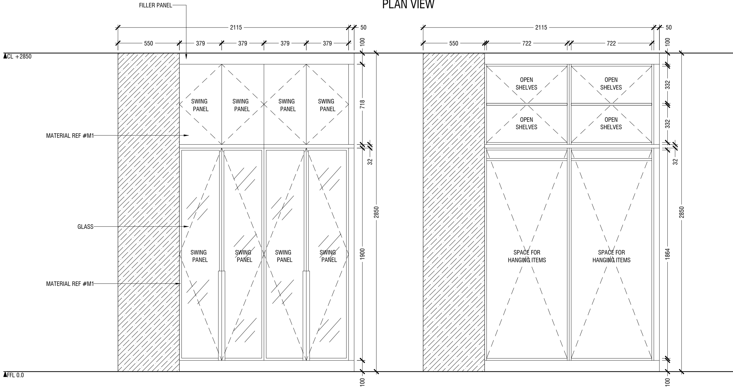
ELEVATION B
