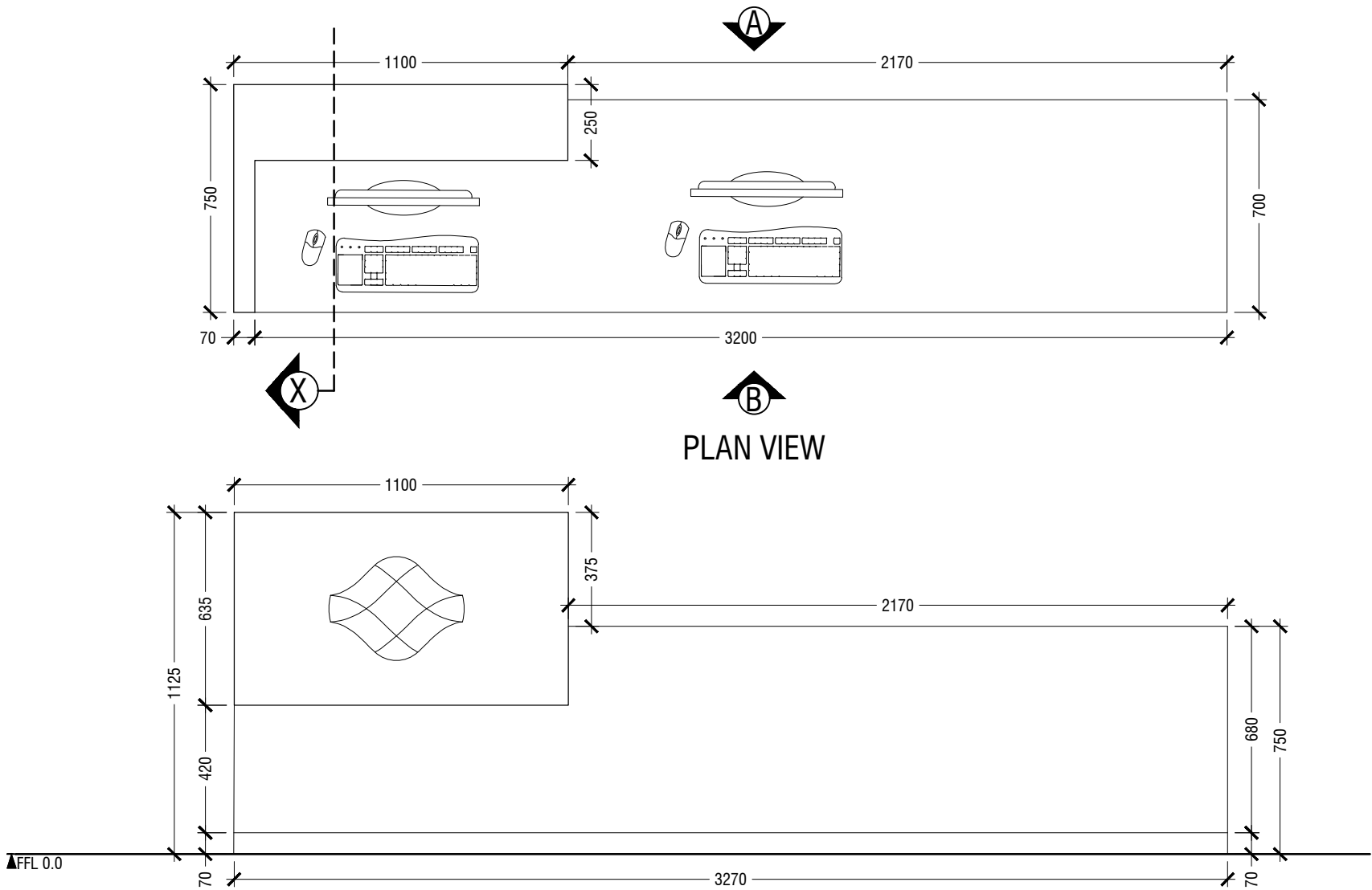
ELEVATION A
