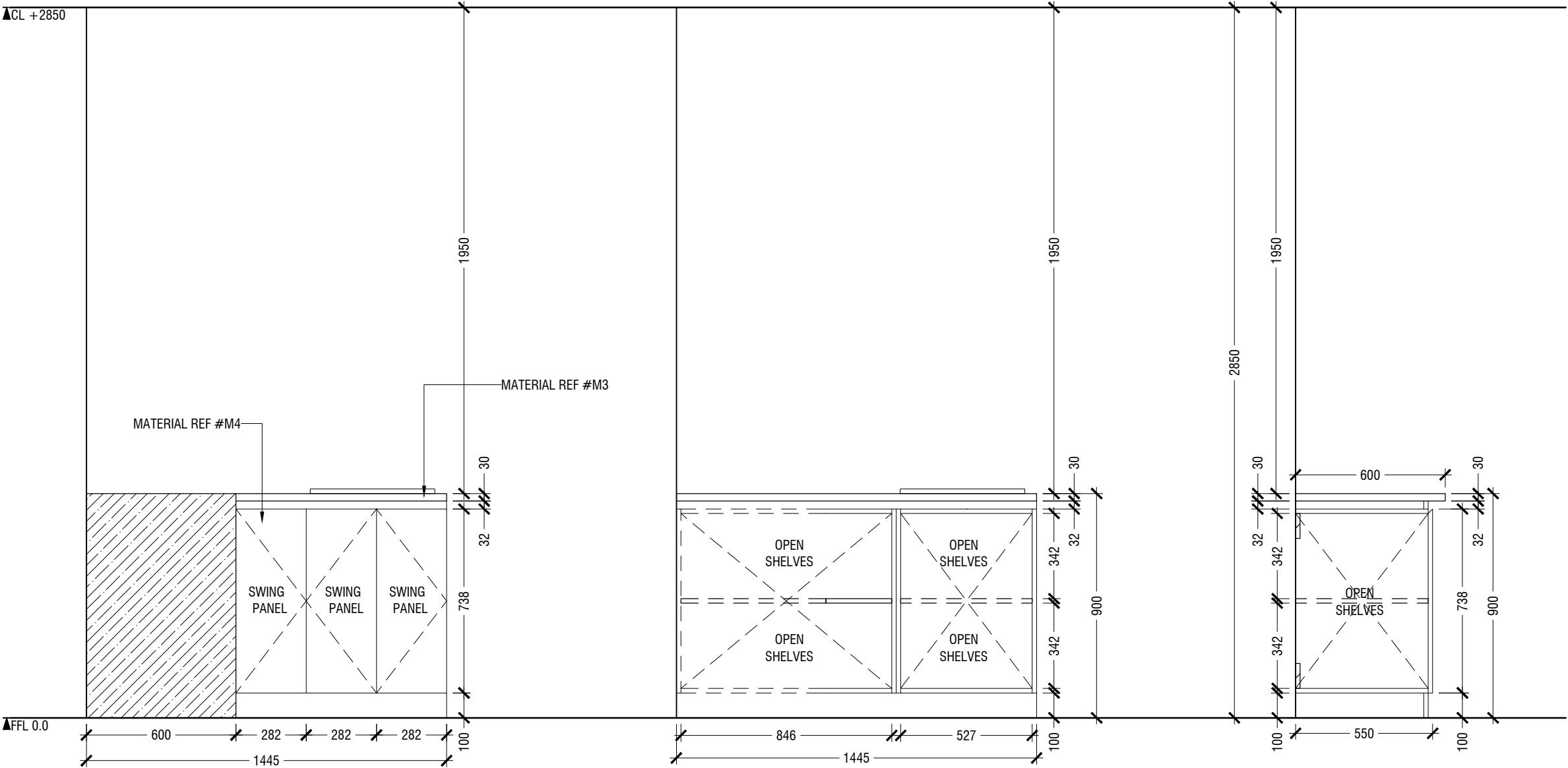
ELEVATION A
