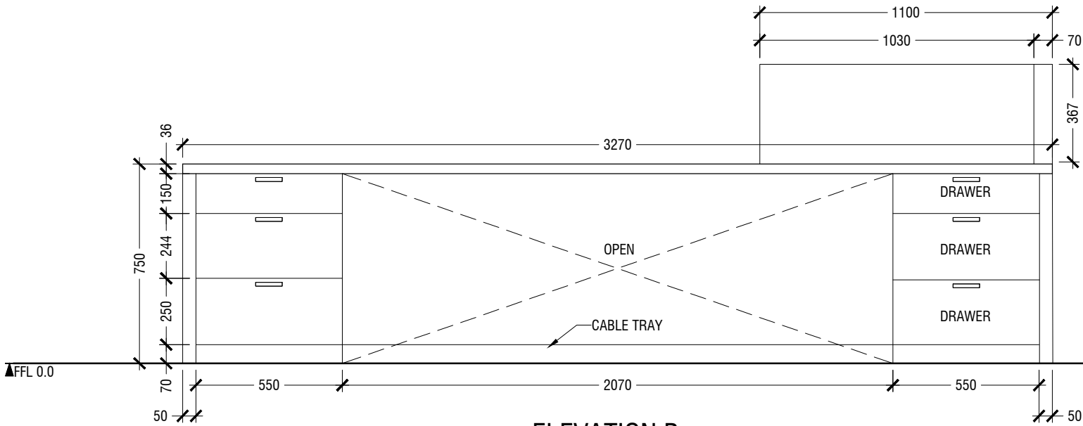
ELEVATION B
