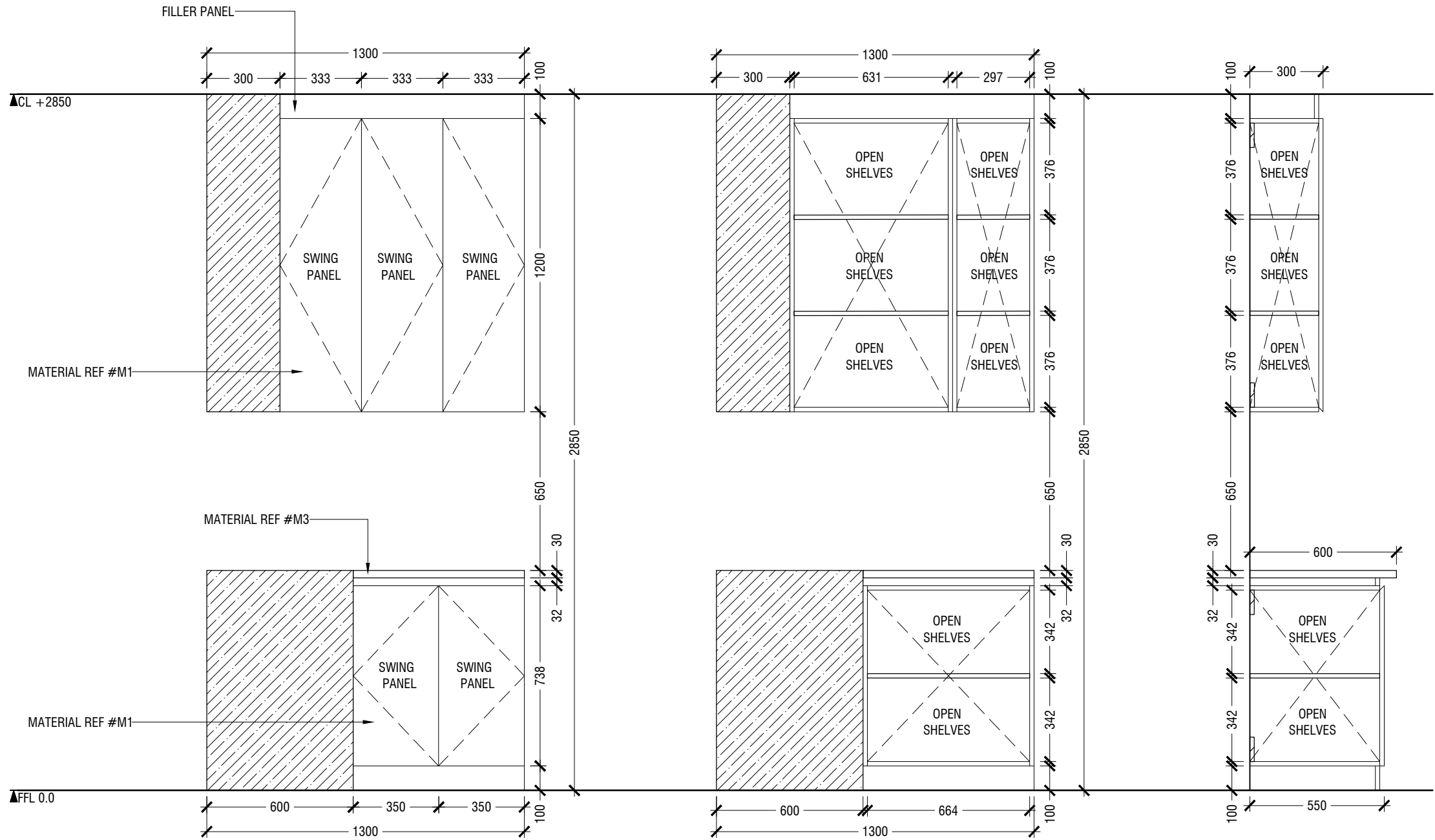
ELEVATION B
